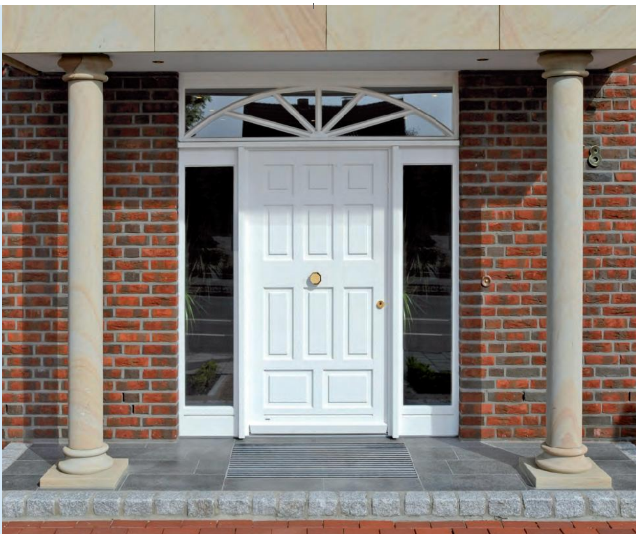
Holz Modell 30351 (PG83/101) Variante: Classic Glas: Klar plan Griff: HA2013 Messing poliert PZ-Rosette: HA7322 Messing poliert mit Kernziehschutz (rund)
