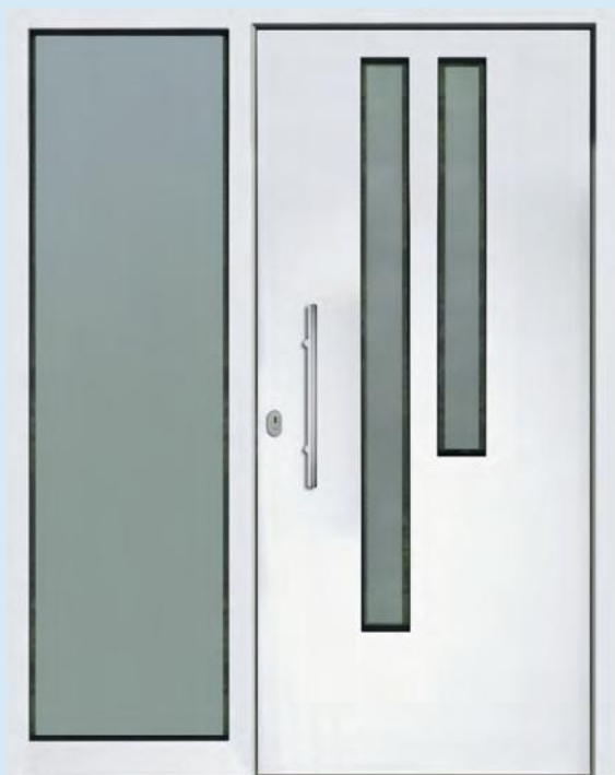
Kunststoff Modell 20457 (PG51) Aluminium Modell 40457 (PG60) Variante: Kontur, mit äußerem Vollblatt-Design 3fach-Glas: Iso klar, Mattierung „Berlin“ Griff: HA1038-60 Edelstahl PZ-Rosette: HA1077 Edelstahl mit Kernziehschutz (oval)
